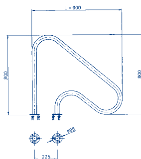
Výstup L = 900
