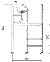
Nárys
