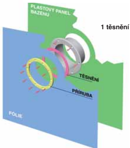
BAZÉN Z PLASTOVÝCH PANELŮ
