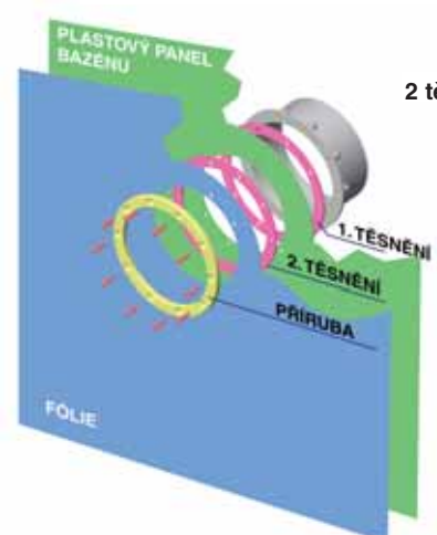
BAZÉN Z PLASTOVÝCH PANELŮ
