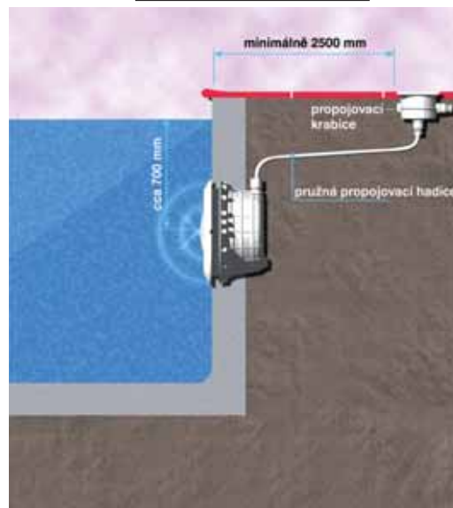
PŘIPOJENÍ TRYSKY NET'N'CLEAN
