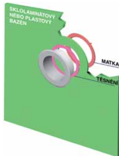
SKLOLAMINÁTOVÝ NEBO PLASTOVÝ BAZÉN
