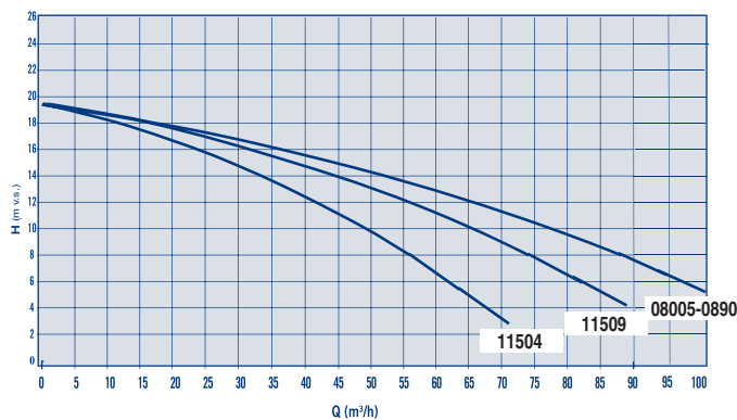
VÝKONOVÉ KŘIVKY ČERPADEL ASTRAL
