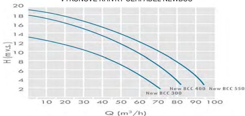
VÝKONOVÉ KŘIVKY ČERPADEL NEWBCC
