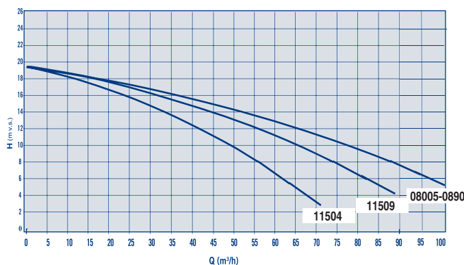
VÝKONOVÉ KŘIVKY ČERPADEL ASTRAL
