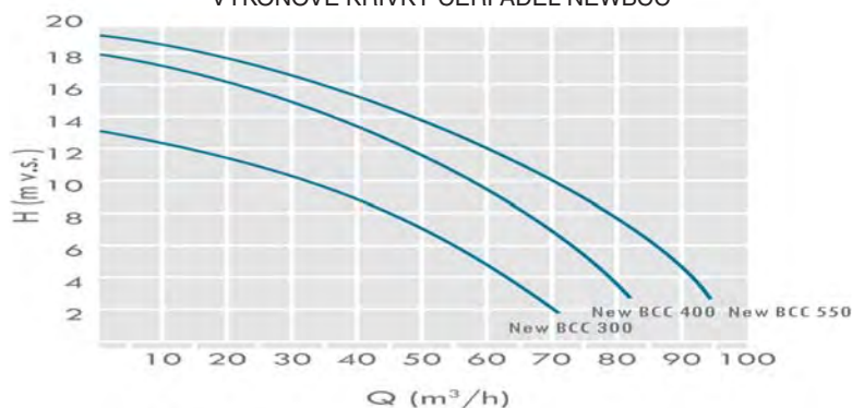
VÝKONOVÉ KŘIVKY ČERPADEL NEWBCC
